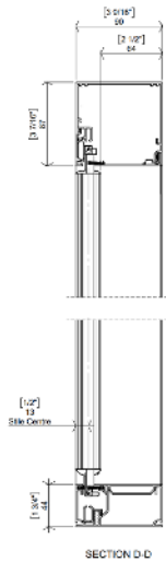
SECTION D-D
